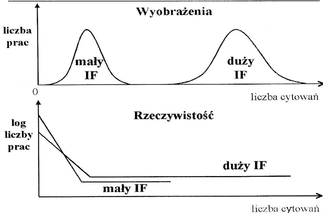
Rys. 11. Rozkład liczby cytowań artykułów w czasopismach o małym i dużym IF
