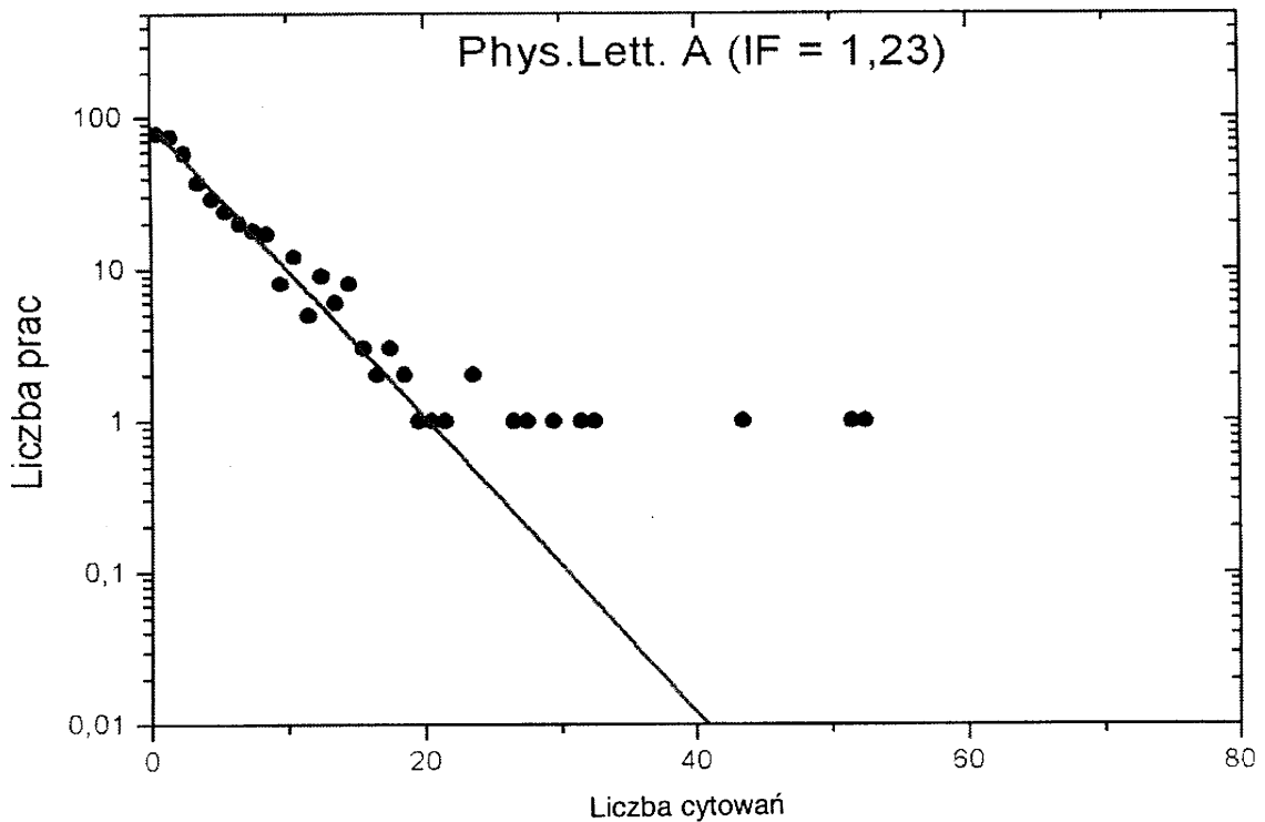
Rys. 14. Rozkład liczby cytowań prac publikowanych w „Physics Letters” A. Linia prosta przedstawia dopasowanie krzywej wykładniczej
