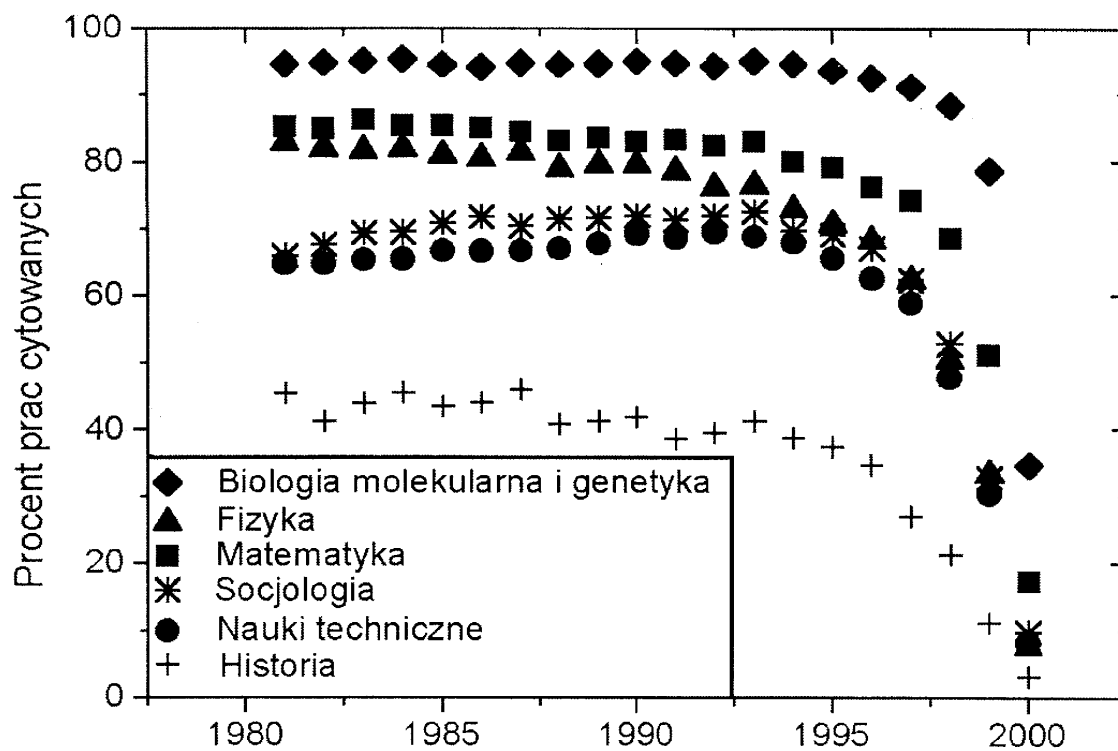
Rys. 24. Procent prac cytowanych w różnych dziedzinach (według bazy NSI 2000)
