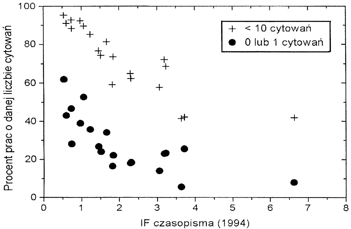
Rys. 21. Procent prac mało cytowanych w zależności od IF czasopisma
