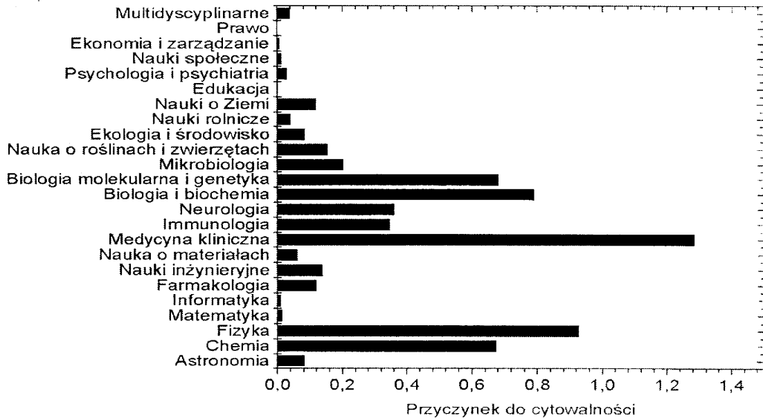
Rys. 7. Wkład do cytowalności różnych dziedzin nauki w Szwajcarii
