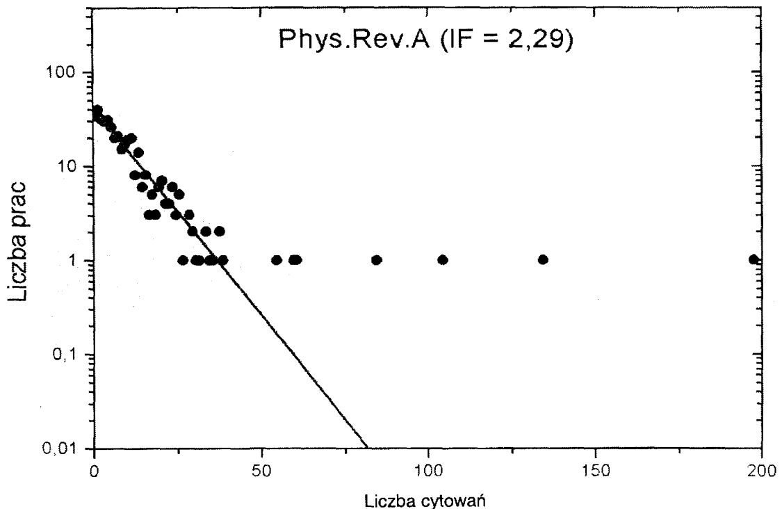
Rys. 16. Rozkład liczby cytowań w „Physical Review”. A. Linia prosta przedstawia dopasowanie krzywej wykładniczej
